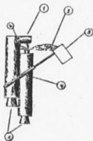
1) Дополнительная трубка, 2) огонь лампы, 3) паяльник, 4) трубка-держатель паяльника, 5) пробка, 6) капсуль.
