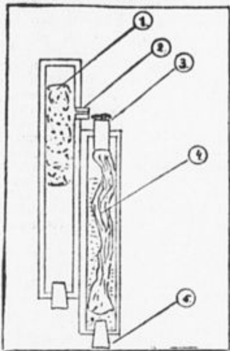
1) Вата, намоченная спиртом, 2) капсуль от примуса, 3—4) фитиль, 5) пробка.
